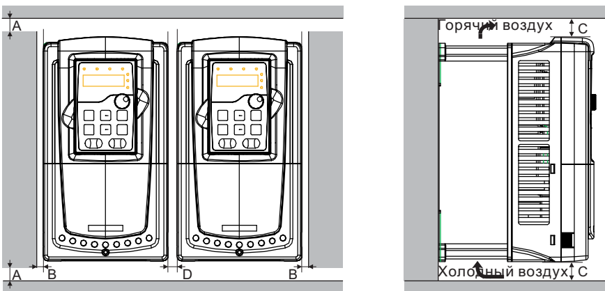
Рис. 4-4 Параллельная установка
