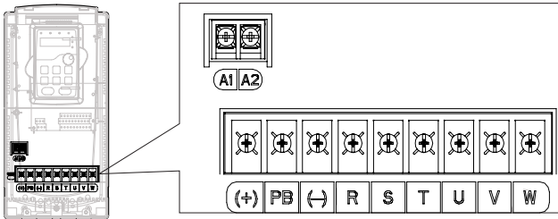
Рис. 4-10 7.5~11 кВ клеммы силовых цепей
